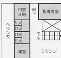
2F平面図
