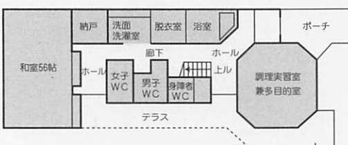
1F平面図
